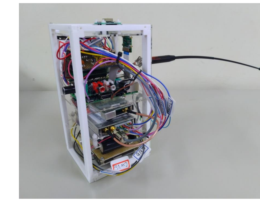
無線通信実験用模型衛星
