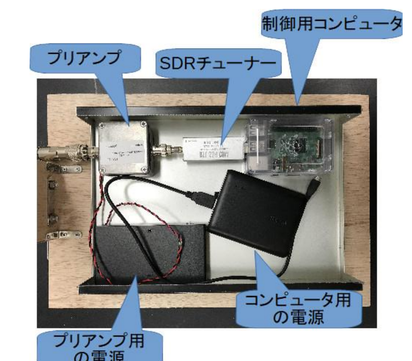
受信機ボックスの構成
